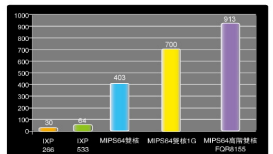
64 Byte小包轉發效能
